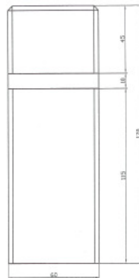
AUFRISS M 1:1
